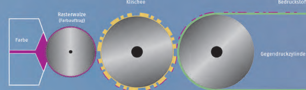
Funktionsweise Flexodruck
